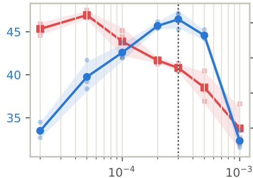
DoRA
