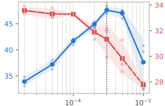
MiLoRA
